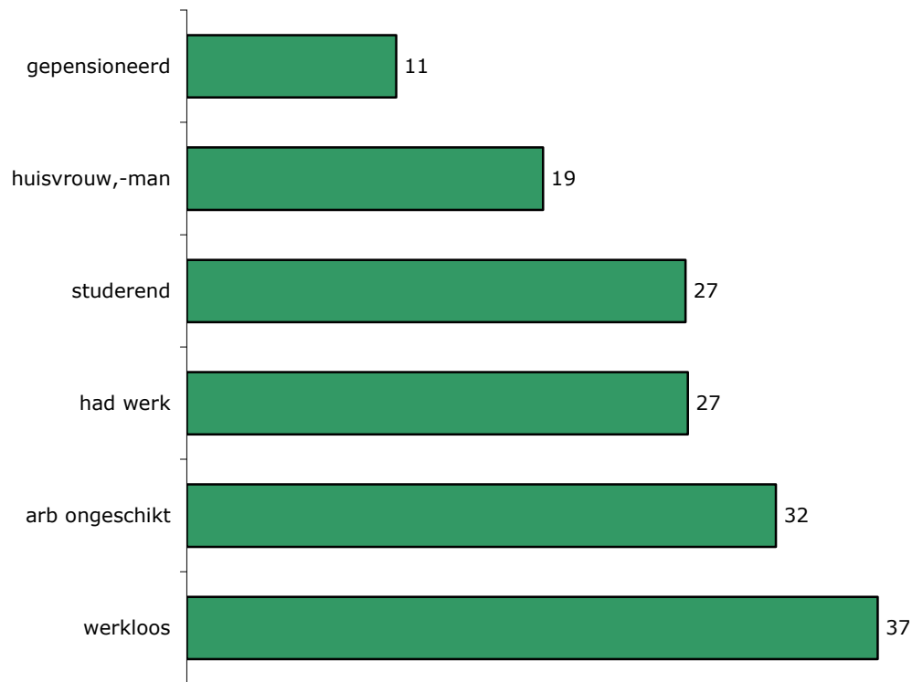
Grafiek 5 Detentierecidive binnen twee jaar na uitstroom naar dagbesteding cohort 2010
