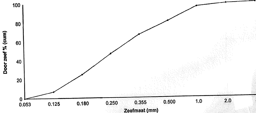
Korrelverdelingsdiagram
