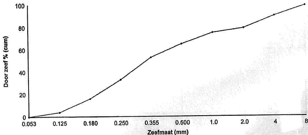
Korrelverdelingsdiagram
