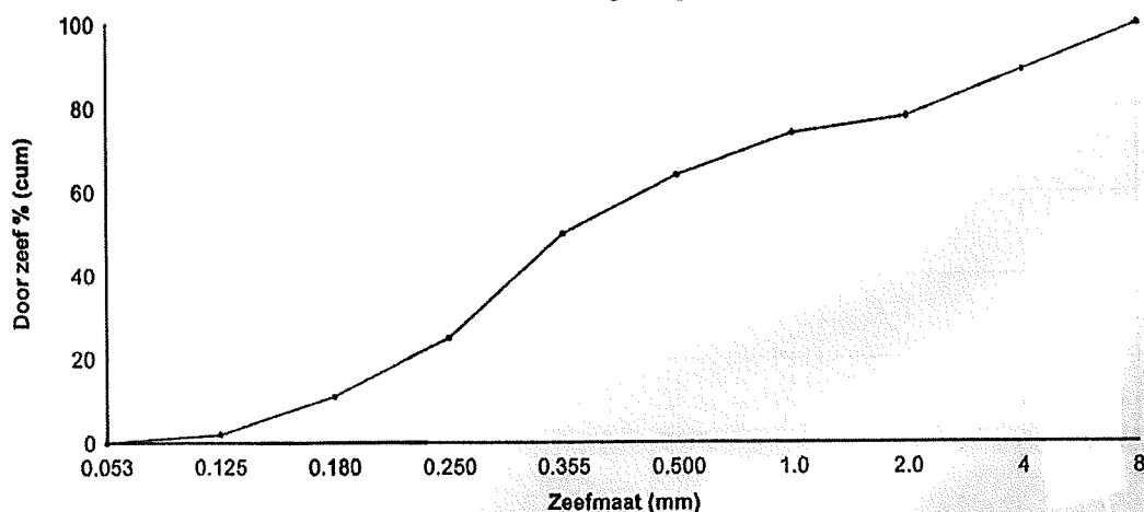
Korrelverdelingsdiagram
